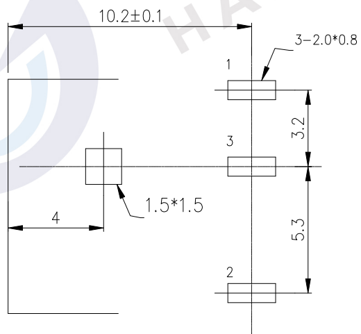
线路板开孔尺寸图
